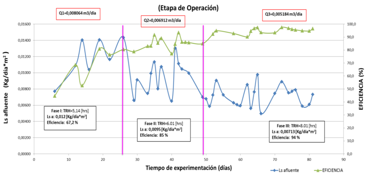
Figura 5. L_s afluente - Eficiencia de remoción vs. tiempo de experimentación
