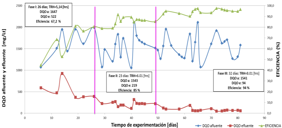
Figura 2. Variación DQO afluente y DQO efluente - Eficiencia vs tiempo de experimentación
