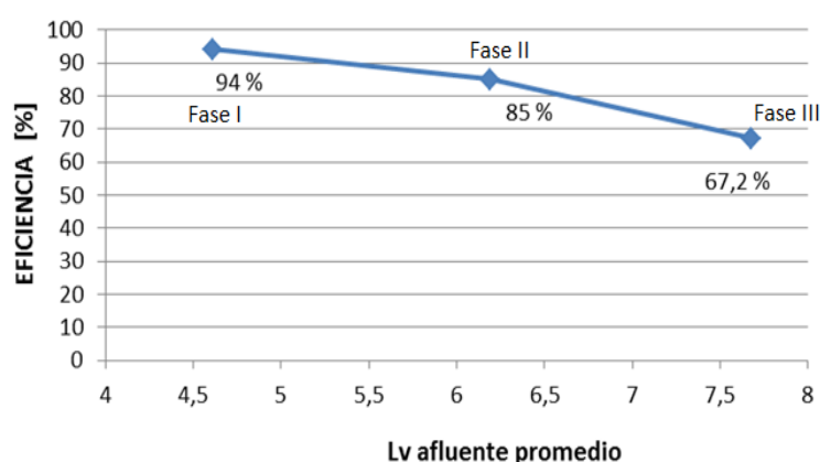
Figura 4. Lv afluente vs. Eficiencia de remoción
