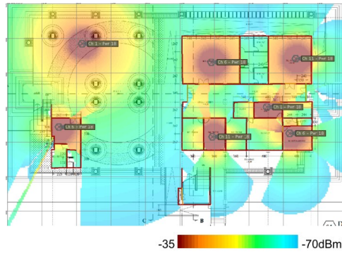
Gambar 16. Peta Sinyal RSSI Lantai 1 JAN
