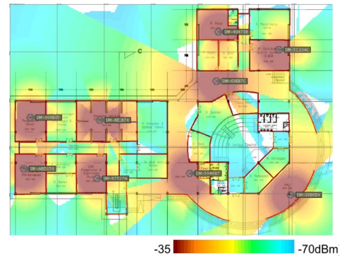
Gambar 11. Peta Sinyal RSSI Lantai 1 JTE
