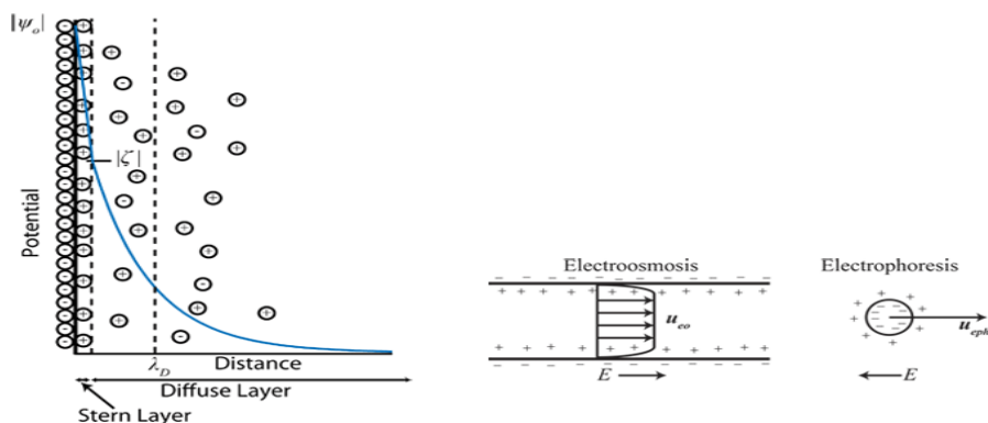
Fig.2 Diffuse layer
