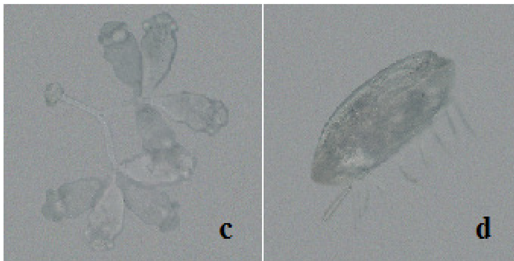
Figura 2 – continuação...Microorganismos encontrados no lodo ativado. (a) Tecameba (Arcella), (b) Rotífero (Philodina), (c) Ciliado Fixo (Vorticella) e (d) Ciliado Livre-Natante (Aspidisca).
