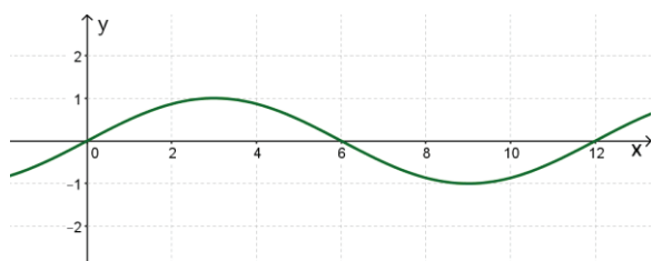
Figura 6: Gráfico da função g
