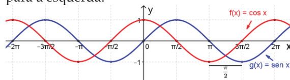
Figura 1: Gráficos das funções f e g
