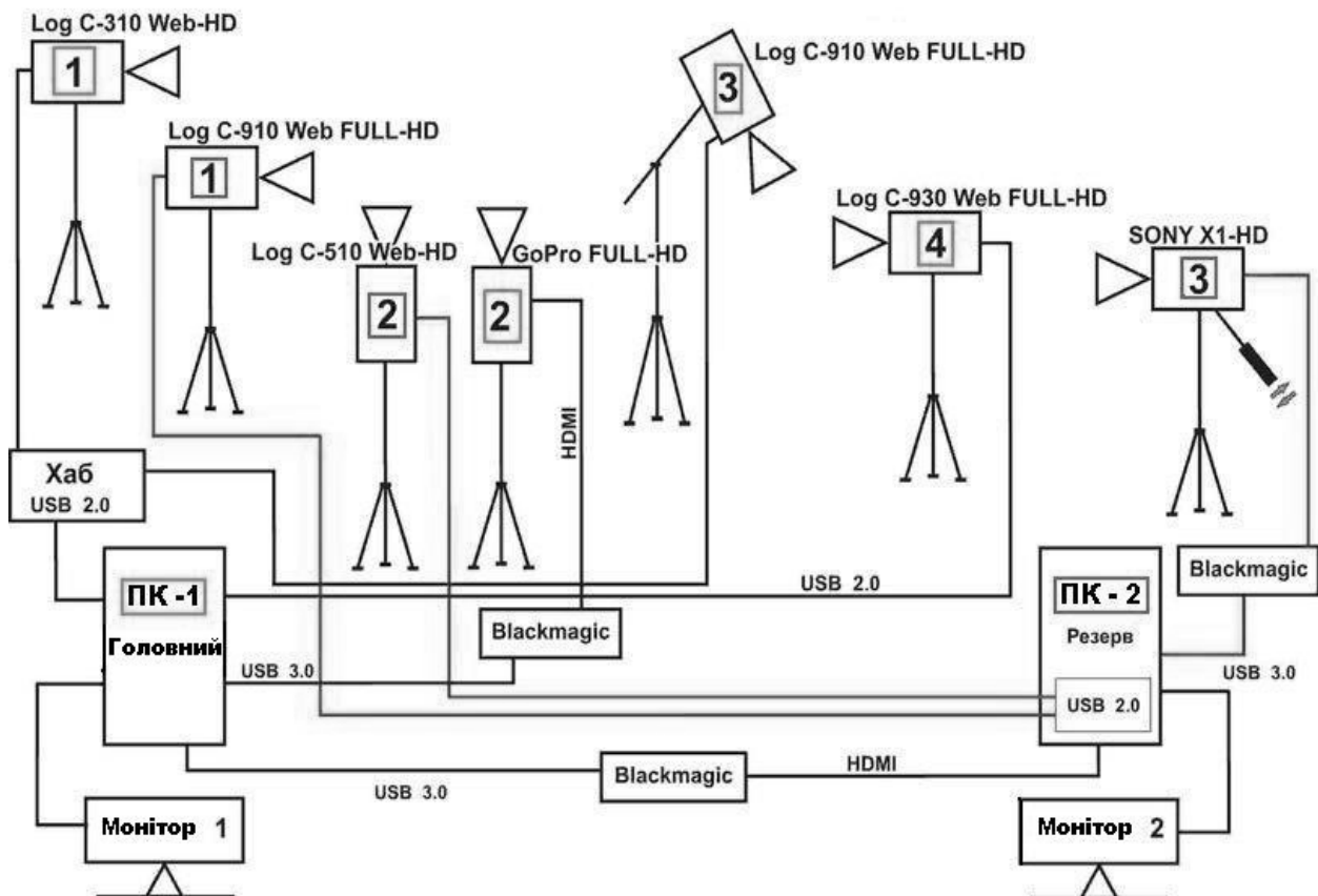
Рис. 2. Підключення та взаємодія камер
