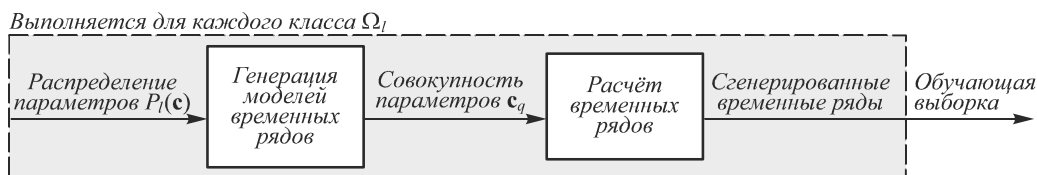
Рис. 5. Генерация обучающей выборки
