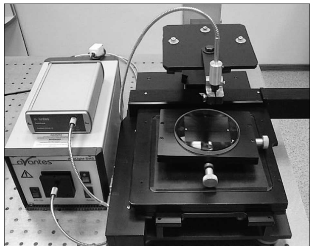
Рис. 5. Экспериментальная установка для измерения глубины травления
