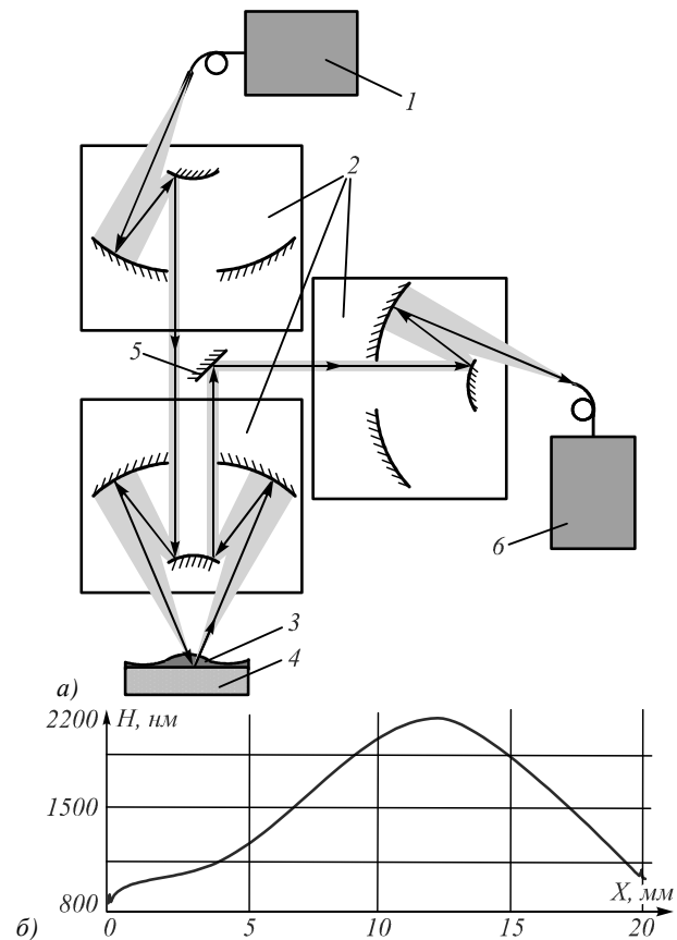
Рис. 9. Модернизированная оптическая схема установки. 1 – волоконный источник света, 2 – зеркальные объективы, 3 – слой фоторезиста, 4 – кварцевая подложка, 5 – поворотное зеркало, 6 – волоконный спектрометр (а).
