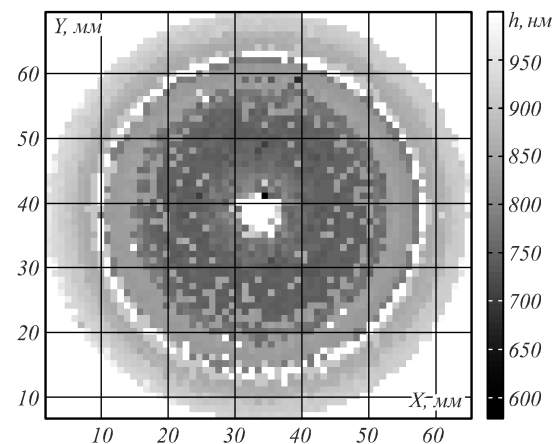
Рис. 6. Карта глубин травления БДОО
