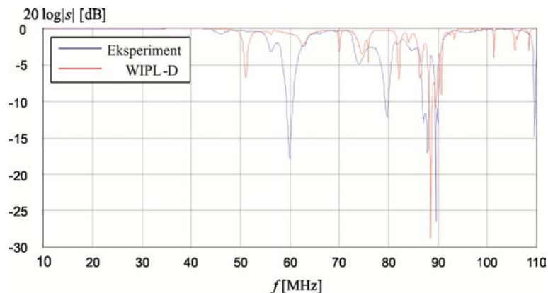
Slika 5 – Modul koeficijenta refleksije kose monopol-antene u kavezu, u funkciji učestanosti, za kavez sa lamperijom
