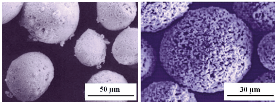
Figure 1 – (SEM) micrograph of the ZrO_2 20\% Y_2O_3 and WC 17\% Co powder particles Slika 1 – (SEM) mikrofotografija čestica praha ZrO_2 20\% Y_2O_3 i WC 17\% Co Рис. 1 – (SEM) микрофотография частиц порошка ZrO_2 20\% Y_2O_3 i WC 17\% Co
