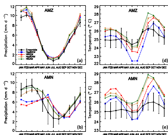
Figura 4 - Ciclo anual da precipitação (mm/dia) e temperatura (°C) nos subdomínios da bacia Amazônica, para as simulações acopladas (linhas pontilhadas) HadGEM (azul) e HiGEM (vermelha) e atmosféricas (linhas contínuas) HadGAM (marrom claro) e HiGAM (verde) e o ensemble de observações (linha preta, a barra indica os máximos/mínimos observados)
