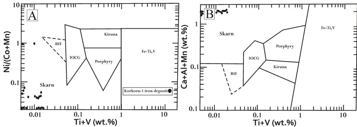
شکل ۱۲. A و B: نمودارهای تفکیک کننده منشأ انواع کانسارهای آهن از (Beaudoin et al., 2007). برحسب آنالیز EPMA اکسیدهای آهن (هماتیت و مگنتیت). طبق این نمودارها، نمونه‌های کانسار آهن کورکورا-۱ در محدوده اسکارن قرار می‌گیرد.
