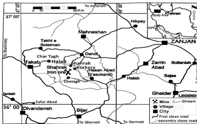
شکل ۲. نقشه راههای دسترسی به معدن آهن شهرک Fig. 2. The access road map to the Shahrak iron mine
