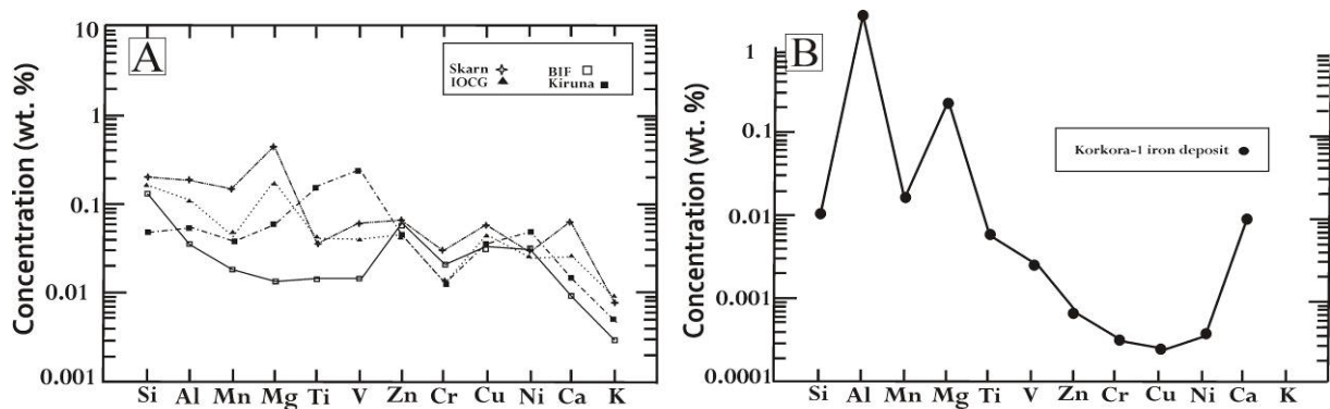
شکل ۱۳. A: نمودار عنكبوتی مربوط به مطالعه انواع کانسارهای آهن بر مبنای غلظت یک‌سری عناصر اصلی و فرعی در کانی مگنتیت و هماتیت از (Beaudoin et al., 2007). B: نمودار عنكبوتی مربوط به نمونه‌های آنالیز میکروپروپوب مگنتیت و هماتیت کانسار کورکورا-۱ که بیشترین انطباق را با تیپ اسکارنی نشان می‌دهد.
