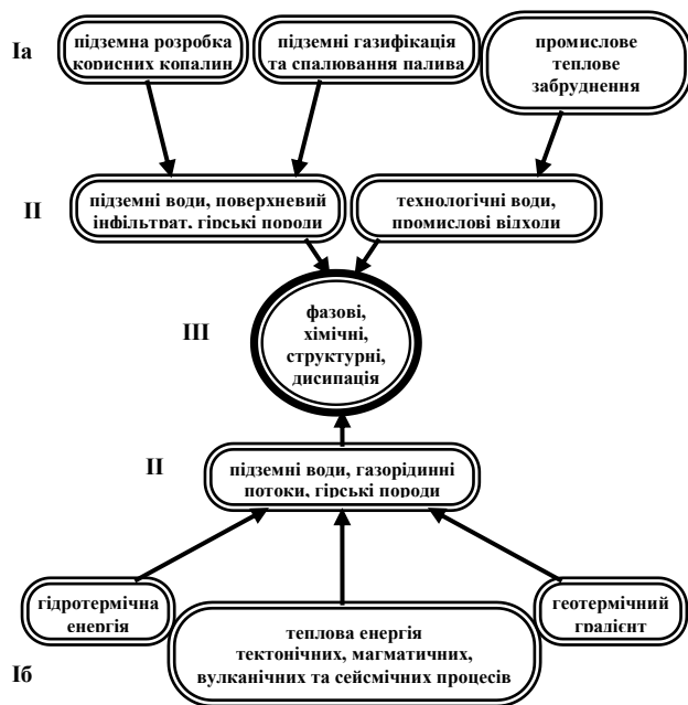
Рис. 1. Схема геотехнічної системи: Ia і Ib – джерела теплової енергії, антропогенні та природні, відповідно; II – шляхи переносу теплової енергії; III – перетворення теплової енергії в геотехнічній системі.
