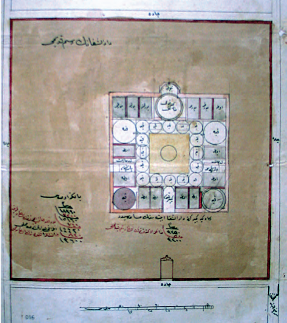
Resim 1. Fatih Darüşşifası Rölöve Planı (BOA)
