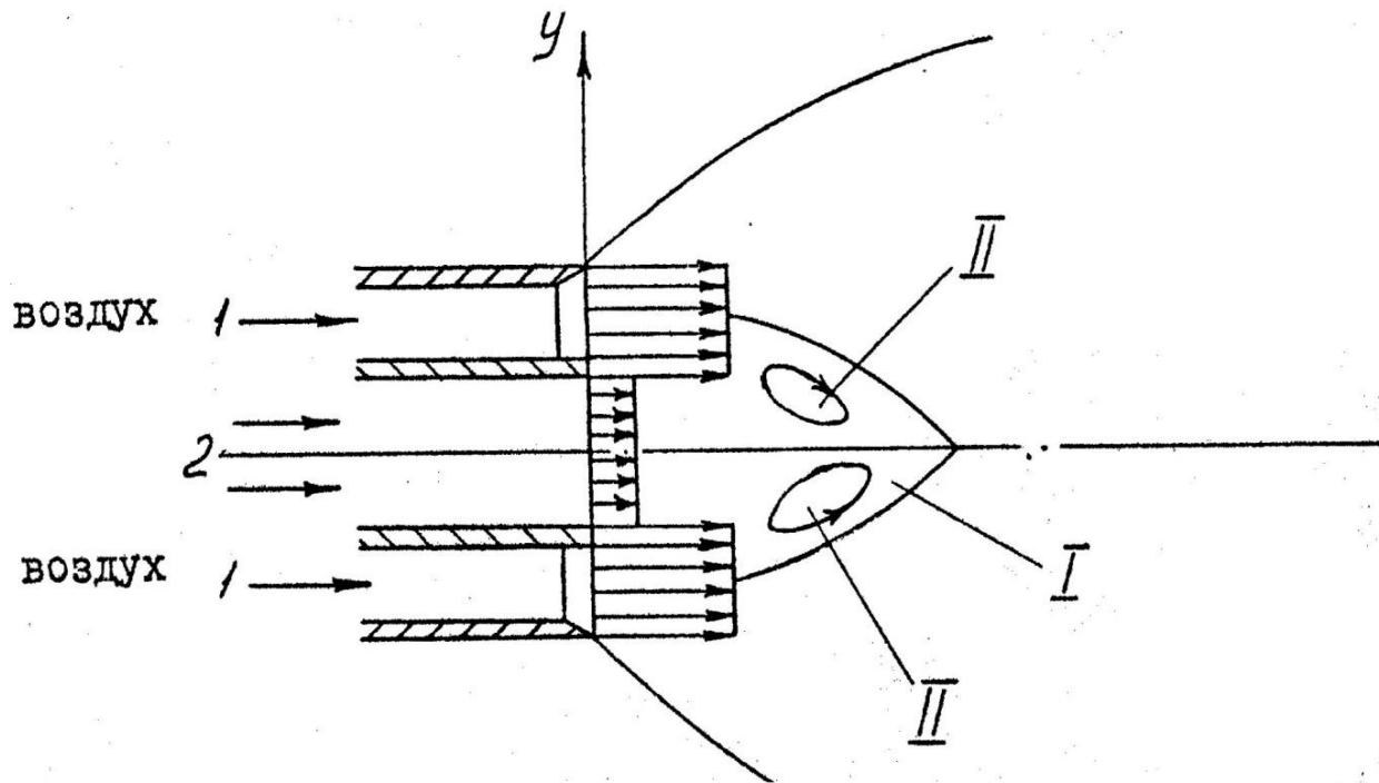
Рис. 1. Схема течения в струе с внутренней зоной разреза в распыляющем рабочем органе
