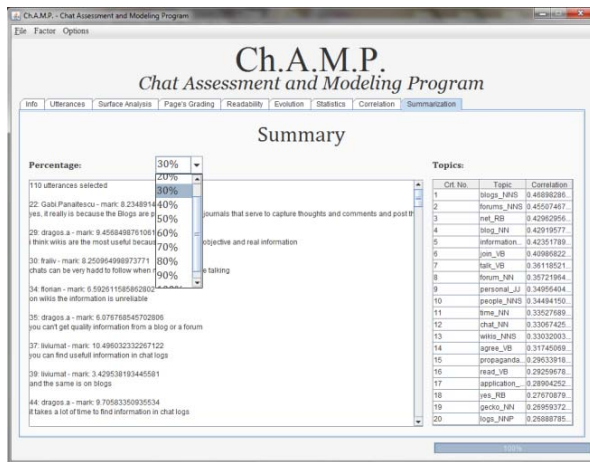
Figura 5. Sumarizare automată
