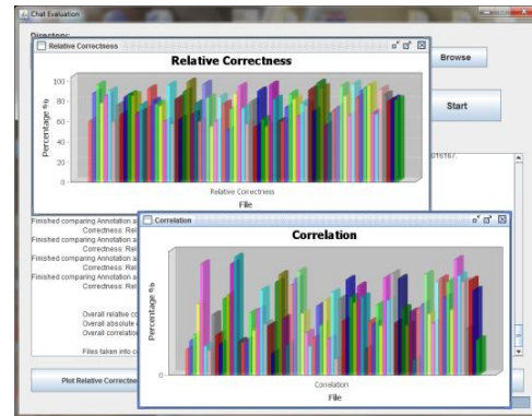
Figura 4. Rezultatele obținute
