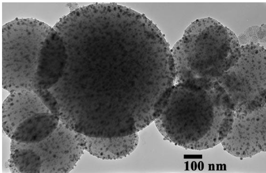
Рис. 2. Электронные микрофотографии мелкодисперстных наночастиц серебра, зафиксированных на поверхности сферических частиц мезопористого алюмосиликата формулы \text{Na}_2\text{O}\cdot\text{Al}_2\text{O}_3\cdot n\text{SiO}_2\cdot m\text{H}_2\text{O} , где n = 1-10 , m = 1-2 [27]
