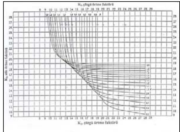
Şekil 6. Love'ın bezayağı örgü için dokunabilirlik sınır grafiği (Love 1954)
