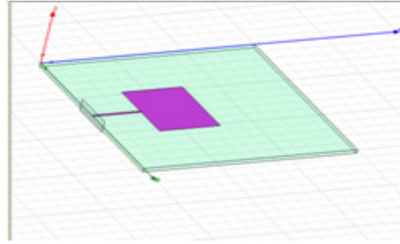
Şekil 2. Tasarlanan antenin HFSS görüntüsü
