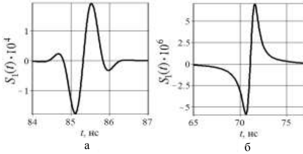
Рис. 4. Форма отраженного сигнала для зондирующего импульса s_1(t) : а – a = 100 см; б – a = 200 см
