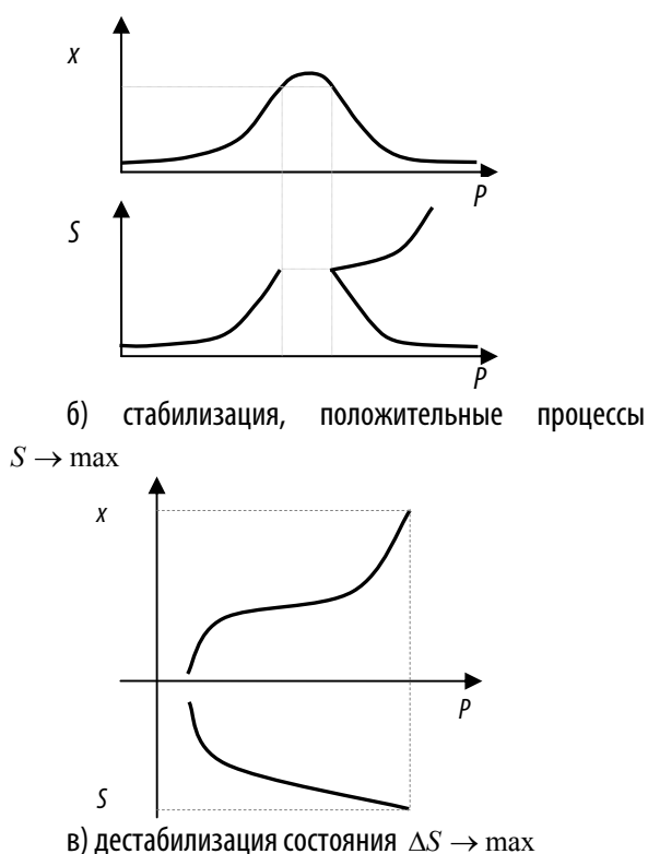
Рисунок 1 – Вероятностно-энтропийная оценка экологичности систем ( P, S и параметр x )
