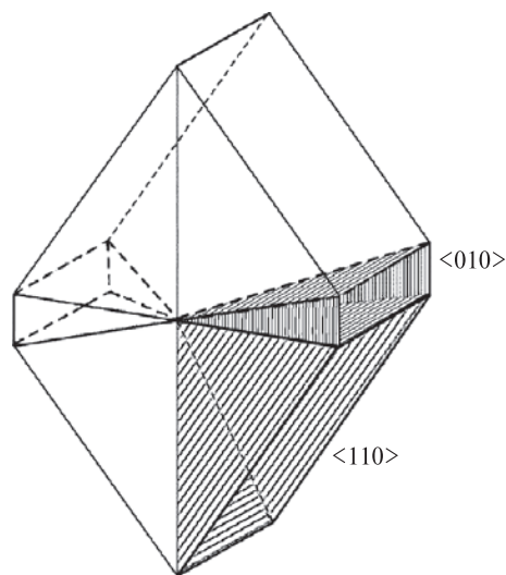
Рис. 1. "Монокристал" топазу з камерних пегматитів Волині. Видно дві різнозабарвлені й різносиметричні піраміди \langle 010 \rangle — блакитна піраміда росту, mm2 і \langle 110 \rangle — рожева піраміда росту, m
