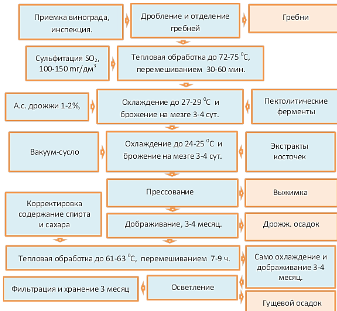
Рисунок 1. Технологическая схема производства специального вина.
