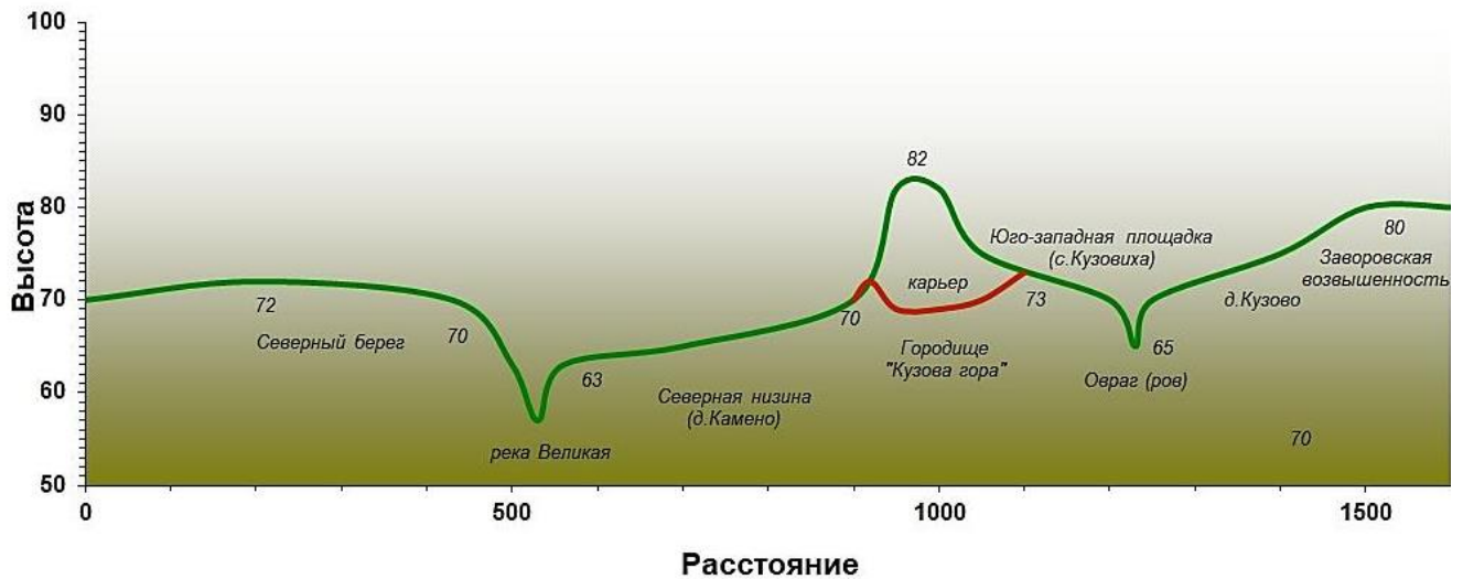
Рисунок 1. Профиль местности через «Кузову гору». (Красным цветом отмечен уровень существующего карьера, зеленым – экстраполяция)
