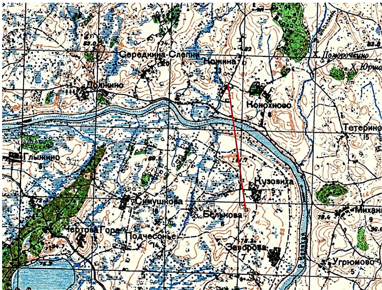
Рисунок 2. Карта окрестностей «Кузовой горы» с линией профиля, представленного на Рисунке 1
