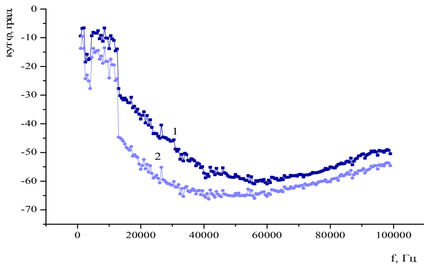
Рис. 3. Фазовий зсув кута \varphi (1 — нативне вовняне волокно; 2 — вовняне волокно після оброблення ТПК)
