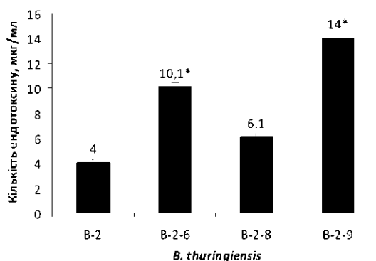
Рис. 2. Кількість \delta -ендотоксину штаму Bacillus thuringiensis В-2 та змінених варіантів:
