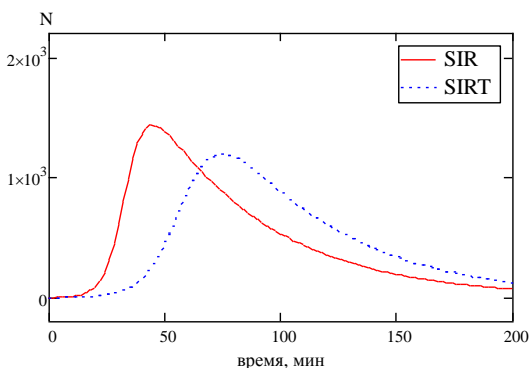
Рис. 2. Графики зависимостей изменения количества зараженных, незараженных и выключенных узлов от времени функционирования компьютерной системы в условиях распространения эпидемии по моделям SIR и SIRT при коэффициенте заражения \beta = 0.25 и частоте лечения \delta = 0.02
