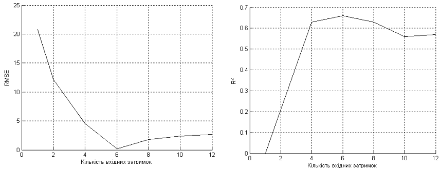
а) за показником якості RMSE
