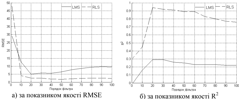
а) за показником якості RMSE б) за показником якості R^2 Рис. 3. Ефективність роботи фільтрів на основі адаптивних алгоритмів RLS та LMS при різному порядку фільтра
