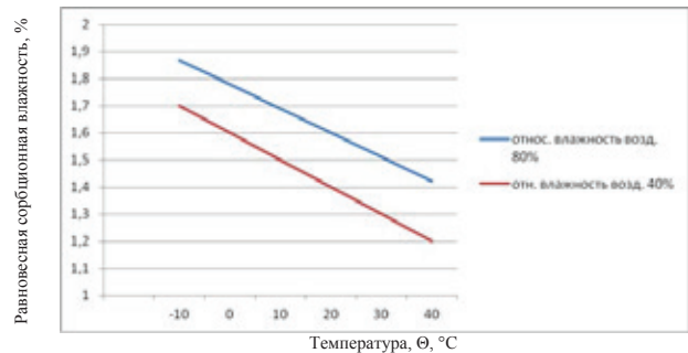
Рис. 4. Зависимость равновесной сорбционной влажности от температуры для ЭППС
