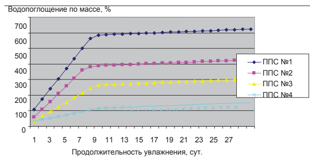
Рис. 5. Зависимость водопоглощения от продолжительности увлажнения пенополистирола: 1- «Новый изодом», 2 – «Изодем», 3 – «СтройПрофи Групп», 4 – «Неомир»
