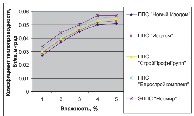
Рис. 1. Зависимость коэффициента теплопроводности пенополистирола от влажности
